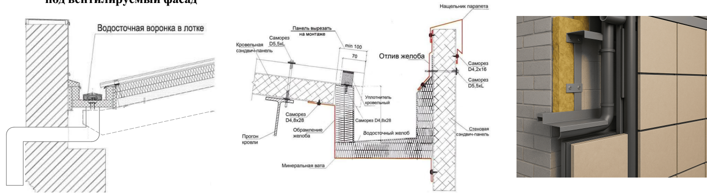
Узлы скрытого водостока под вентилируемый фасад
